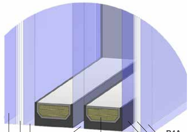
P4A 4mm klaas 4 teipi 4mm klaas Soojustatud distantihoidik 12–36mm P4A 4mm klaas 4 teipi 4mm klaas
